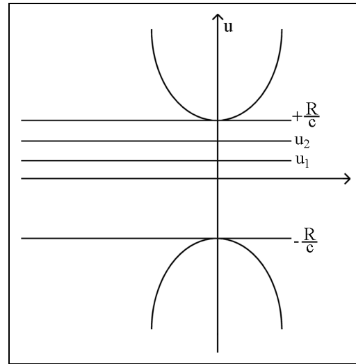
Abb. 14: Kleinsche Deutung affin skizziert
