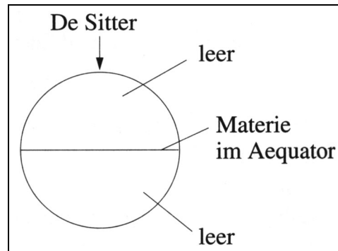
Abb. 11: Äquatorialer Massenring
